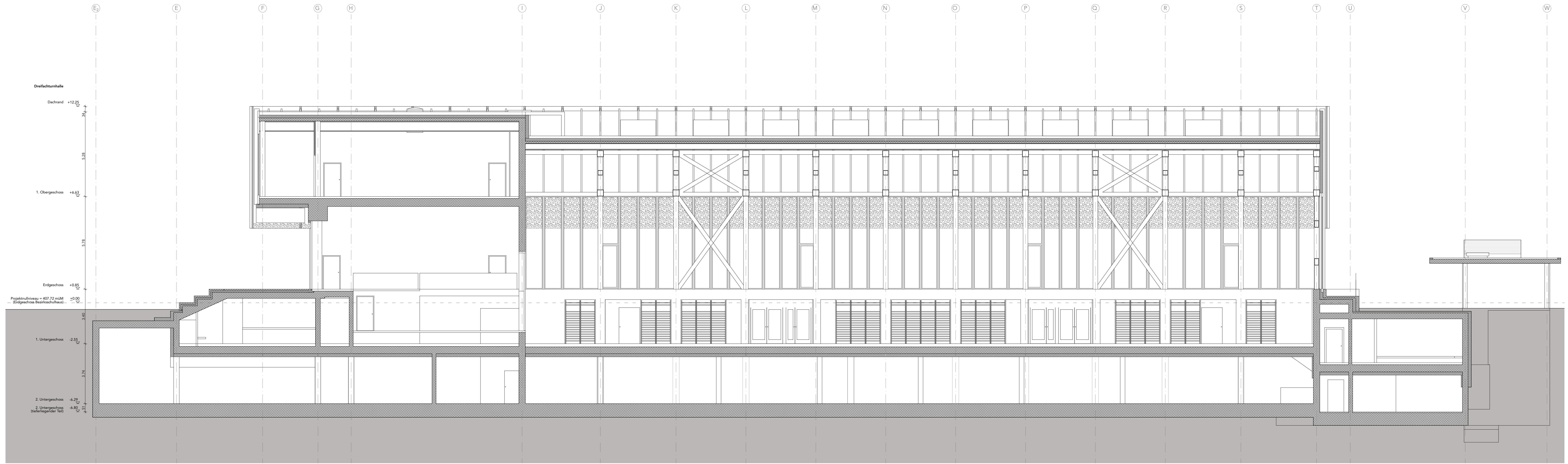
Schnitt 1
