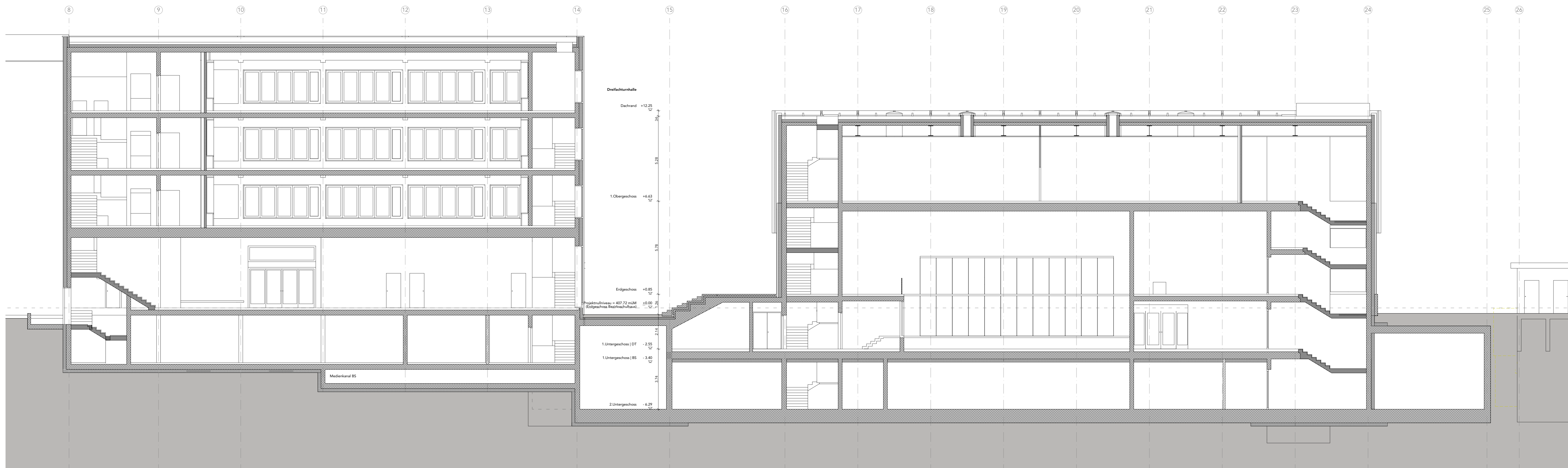
Schnitt 5
