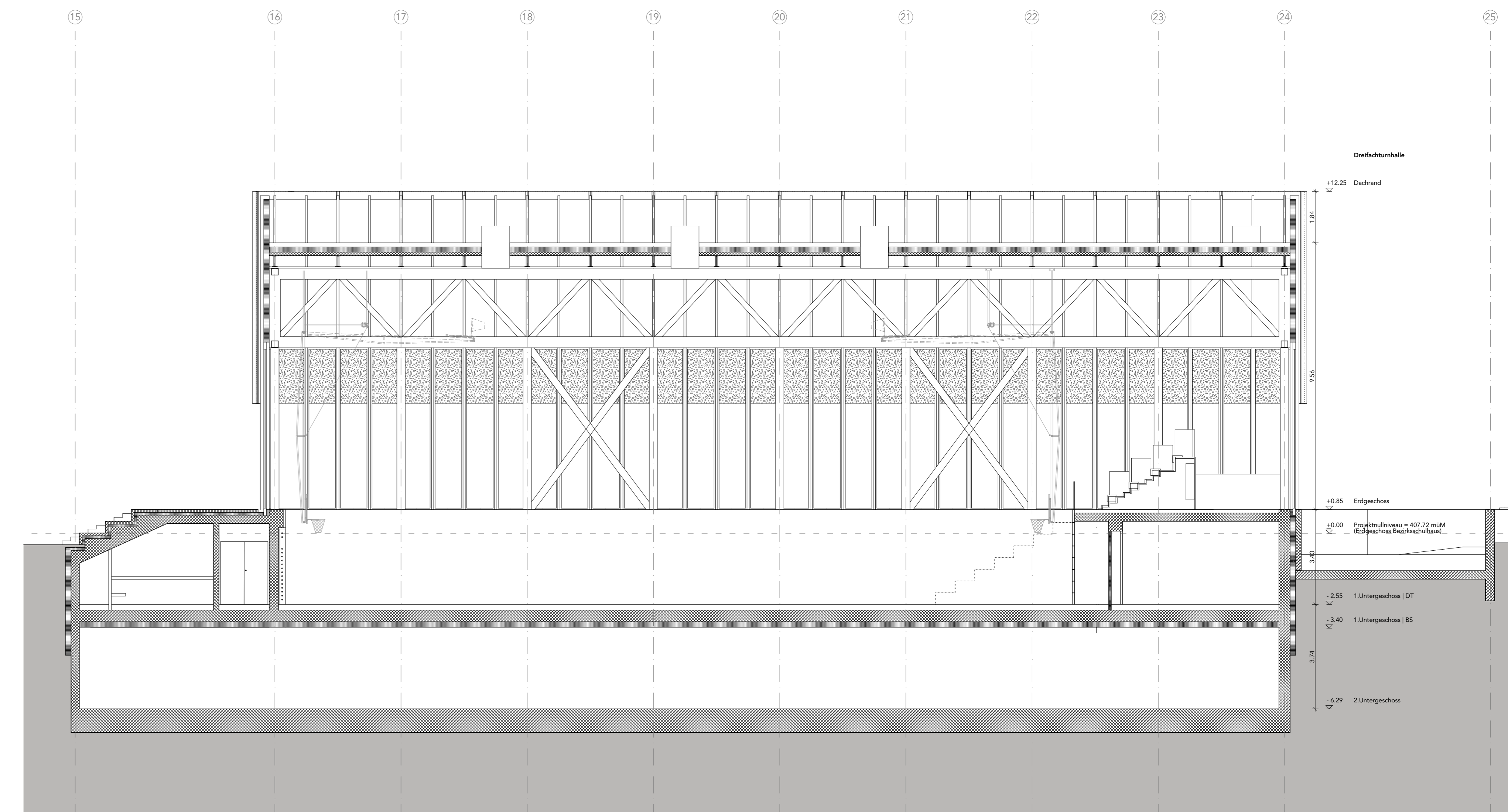
Schnitt 4
