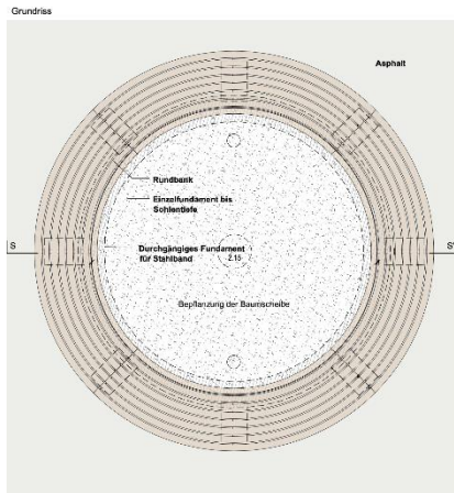
RD-106, Baumscheibe offen mit Rundbank
